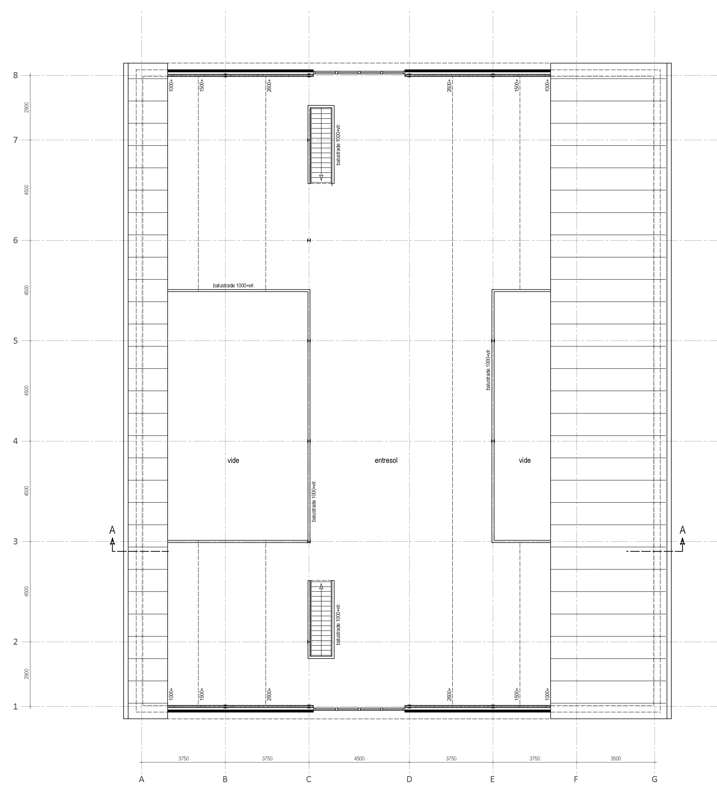
verdieping bestand
