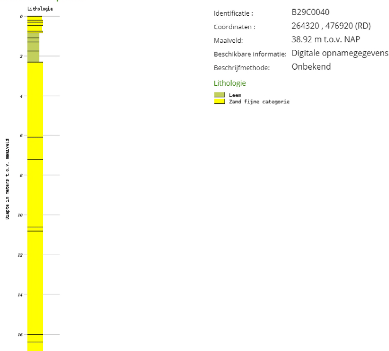
Afbeelding 2.1: Boorbeschrijving boring B29C0040 (bron: Dinoloket)
