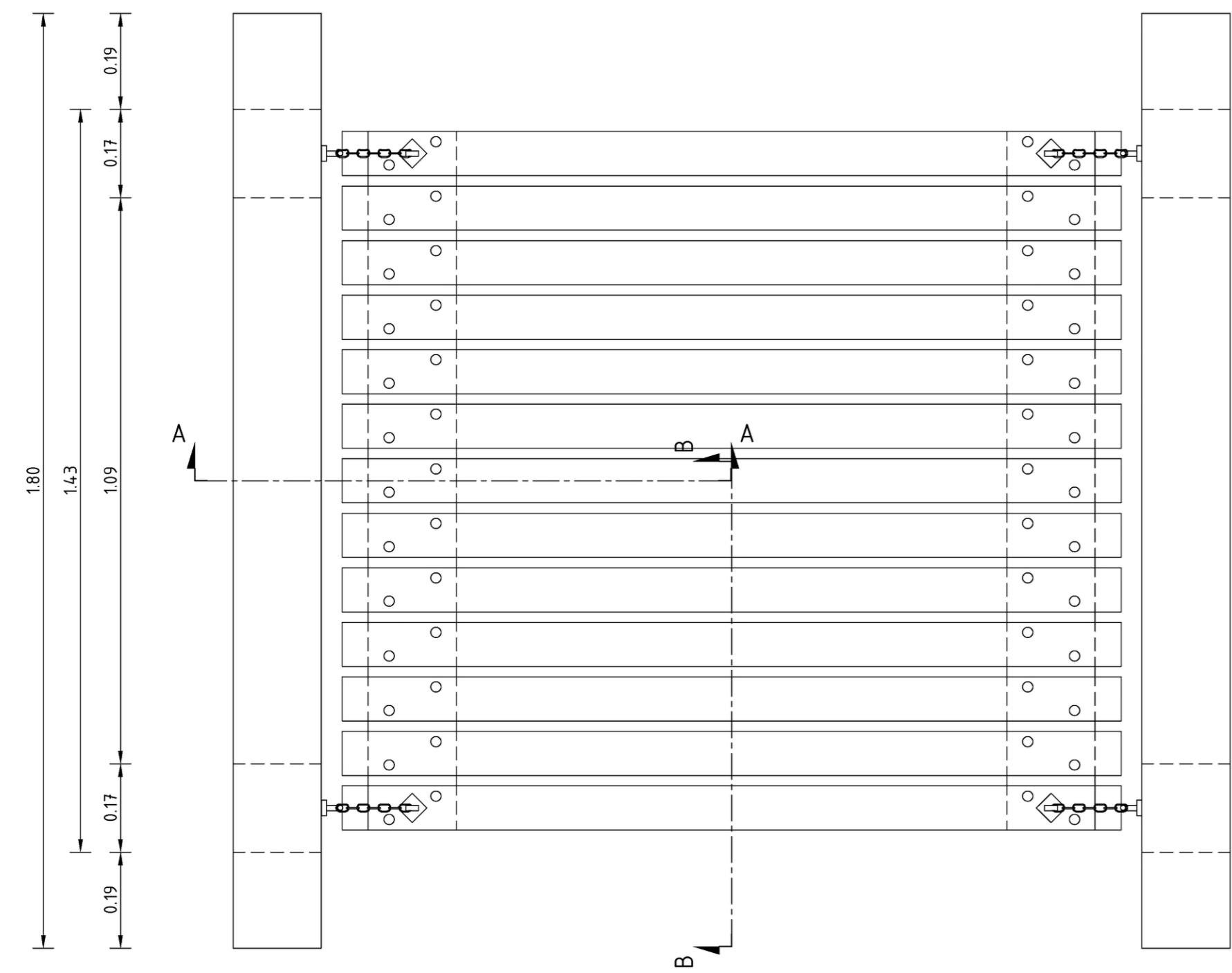
Bovenaanzicht Schaal 1/10
