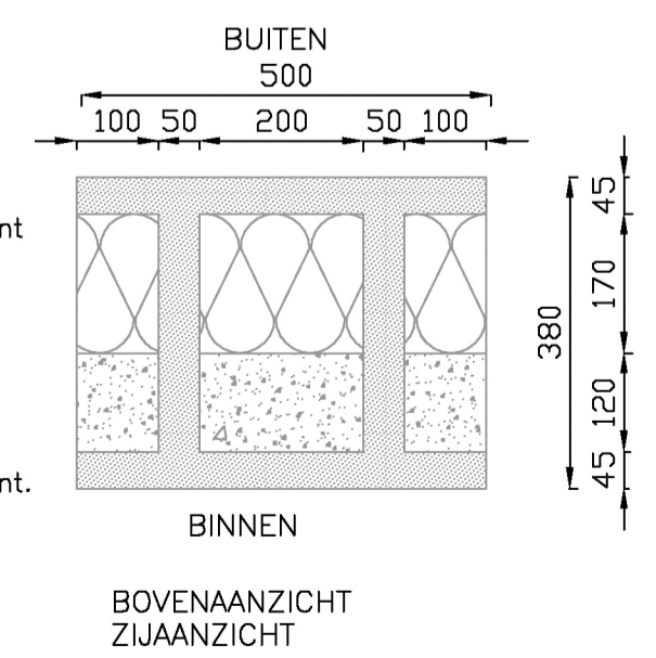
BLOKPRINCIPE 1:10
