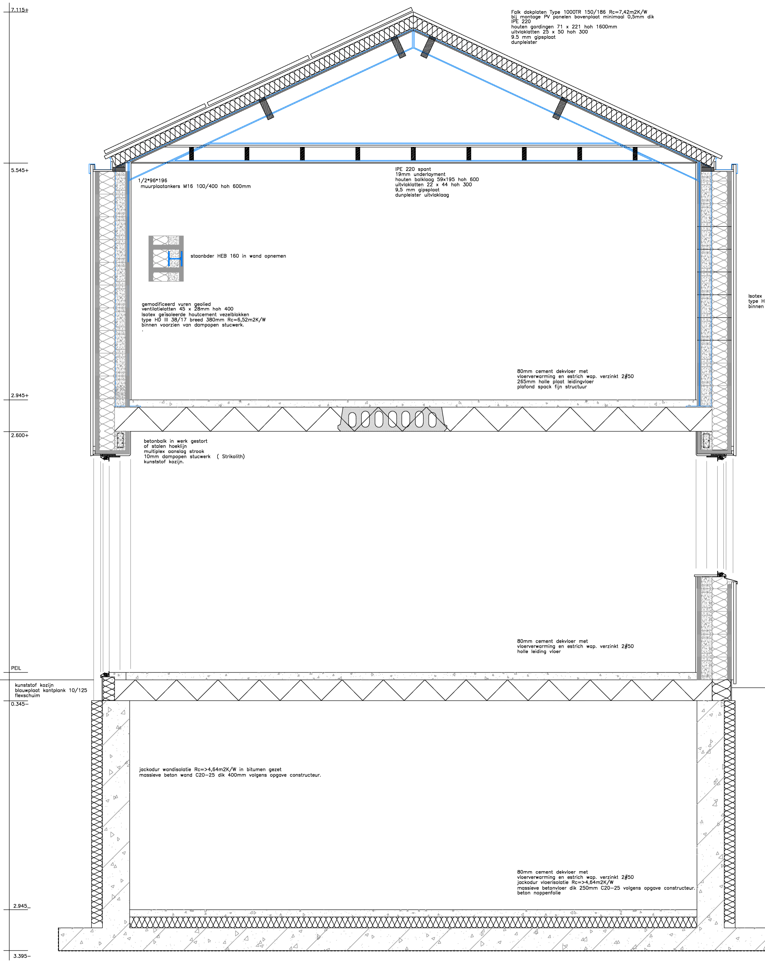
DOORSNEDE over hoofdbouw
